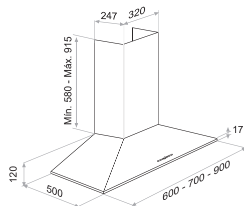
Dimensions en / Dimensions in mm Tubes spéciaux personnalisés / Special custom-made chimneys
