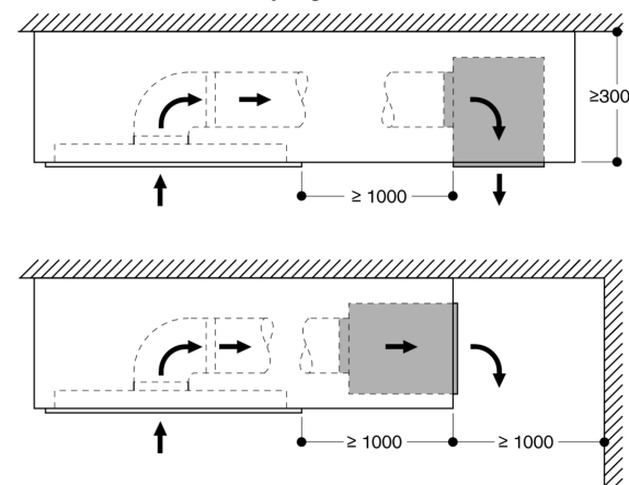
Mesures en mm
