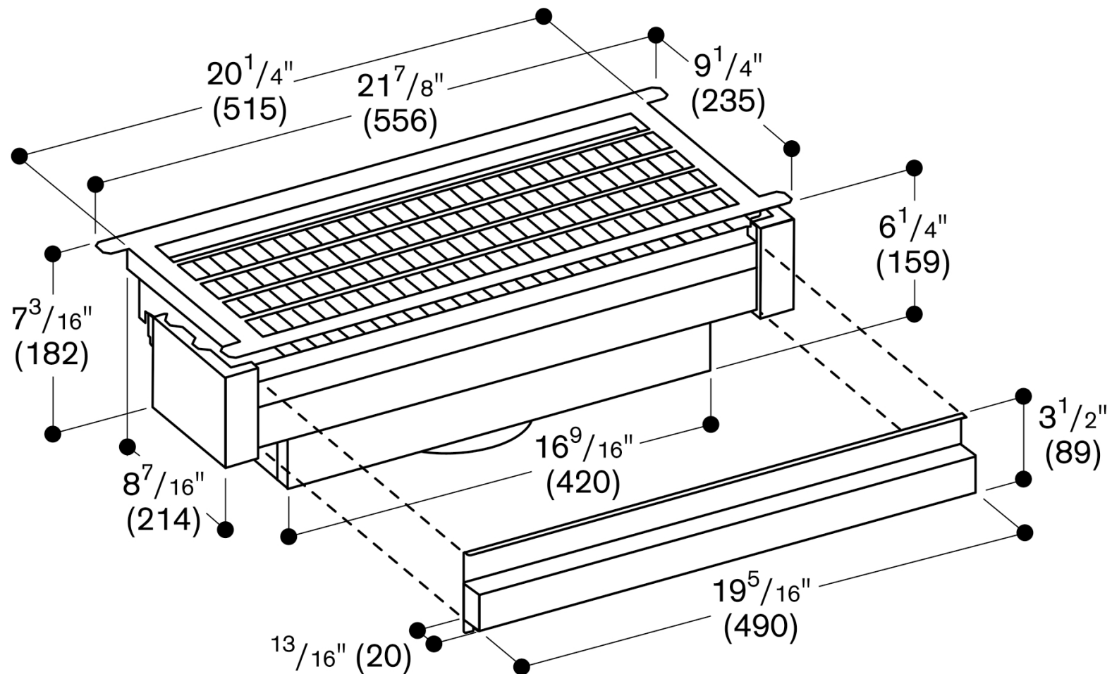
Couvercle de filtre amovible
