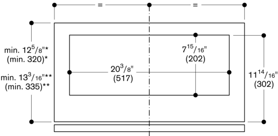
Vue du meuble haut du dessus avec AA 211 812
