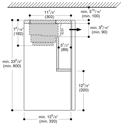
Section transversale du meuble haut avec AA 211 812
