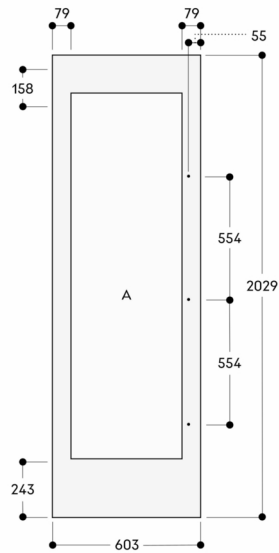
Largeur de niche 610 mm
