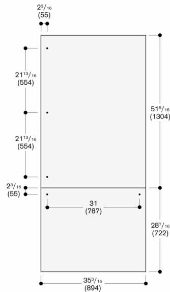
Largeur de la niche 35,5" (900 mm)
