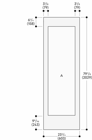
Largeur de niche 24" (610 mm)
