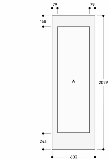
Largeur de niche 610 mm
