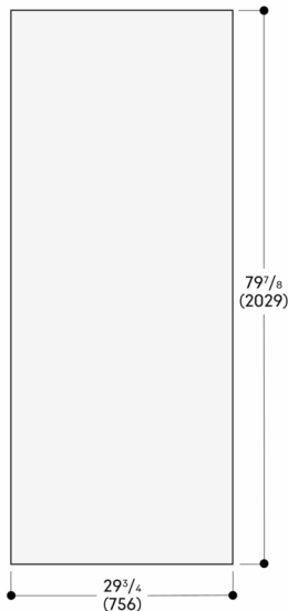
Largeur de niche 30" (762 mm)
