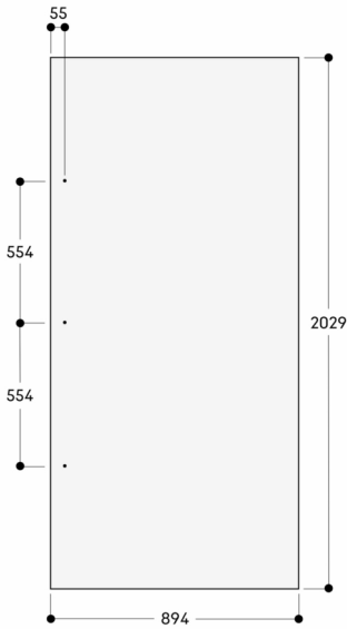
Le panneau d'habillage fait 19 mm d'épaisseur Les dimensions maximales des panneaux d'habillage sont basées sur un jeu de 3 mm, sur la base d'une seule niche Mesures en mm
