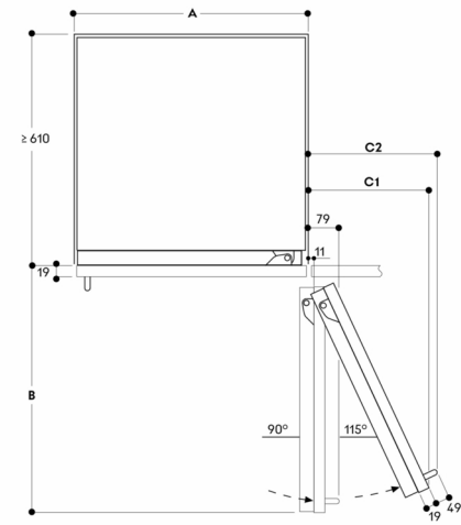
Distance au mur RVB/RVC/RVF/RVW
