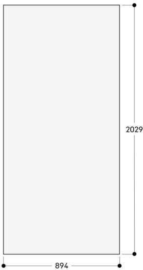
Le panneau d'habillage fait 19 mm d'épaisseur Les dimensions maximales des panneaux d'habillage sont basées sur un jeu de 3 mm, sur la base d'une seule niche Mesures en mm
