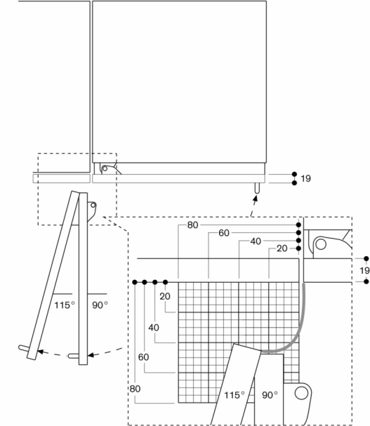
Angle d'ouverture de porte
