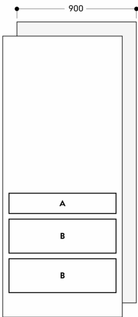
A: Tiroir fraîcheur B: Tiroir fraîcheur avec contrôle de température et d'humidité Mesures en mm
